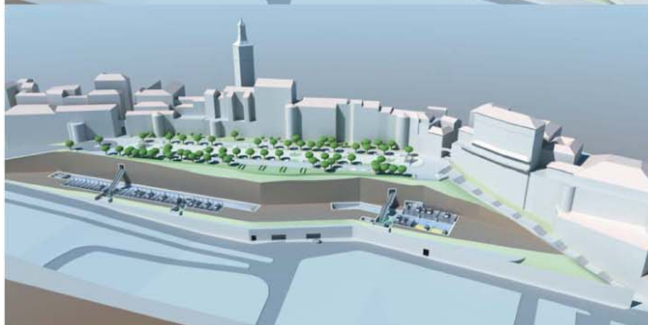
Nivel 2. Aparcamiento de residentes. 89 plazas
